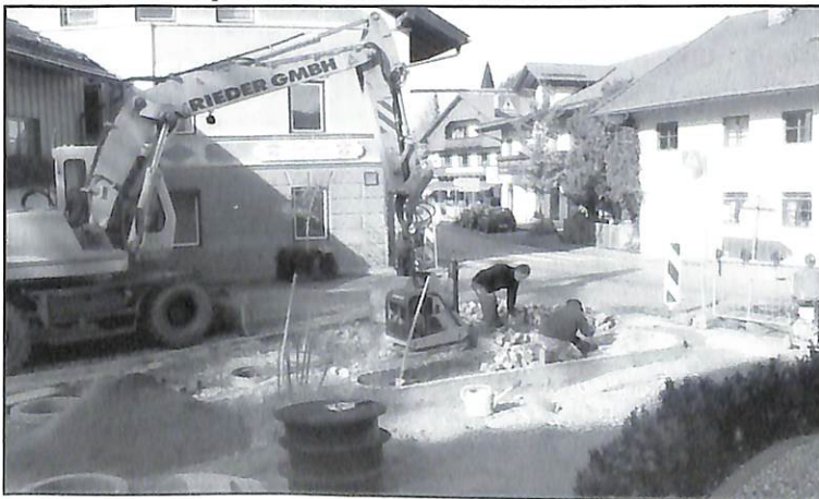
Das Sonderbauwerk an der Einfahrt zur Haslacher Straße ist fertig.
