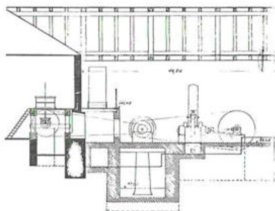
Schnitt senkrecht zur Kanalaxe
