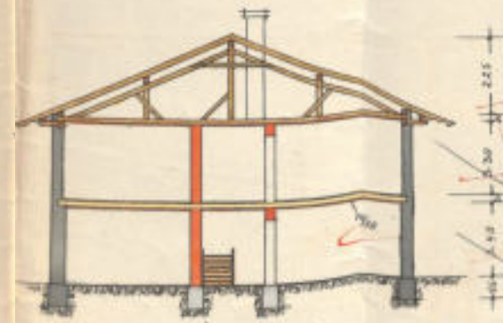
Schnitt A-B
