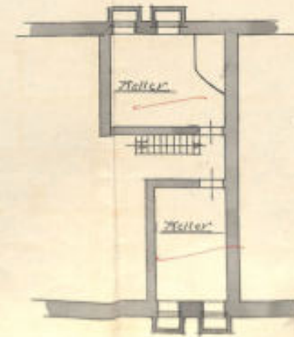
Keller Grundriss
